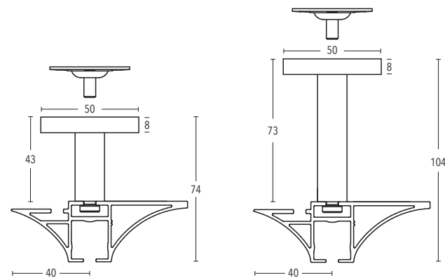
Ceiling bracket 43 mm and 73 mm art. no. 11473-50 und 11473-80
